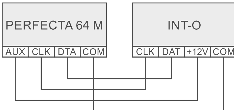
Rys. 13. Podłączenia ekspandera INT-O do centrali.
