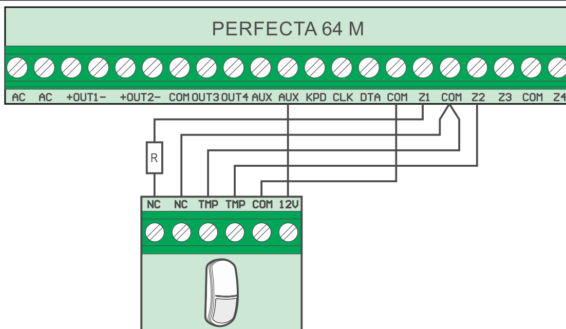
Rys. 21. Przykład podłączenia czujki NC w konfiguracji EOL.
