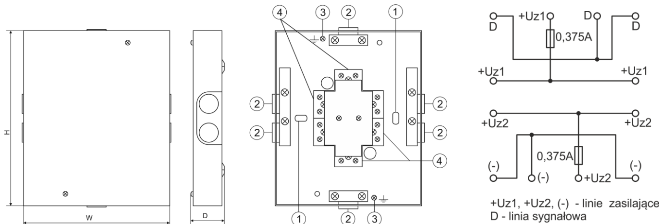
Rys.1. Widok puszki instalacyjnej i schemat połączeń.
