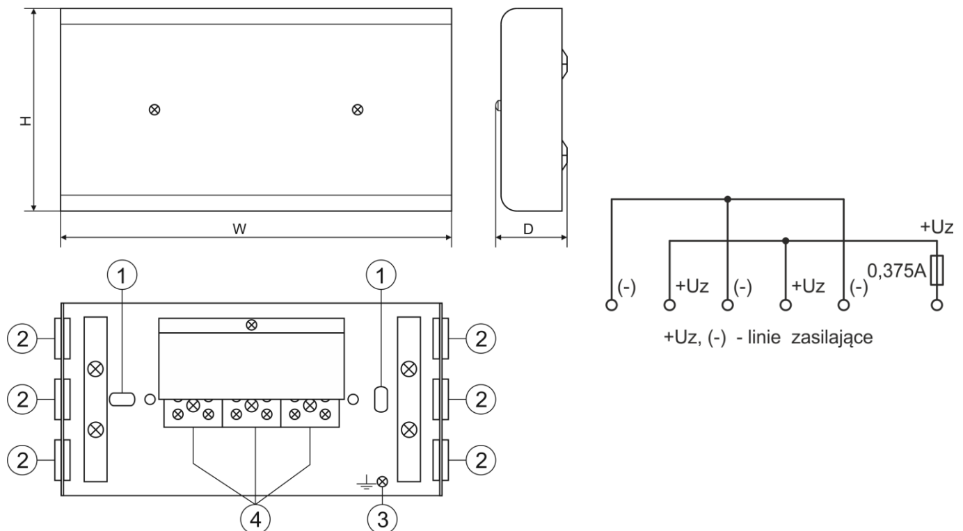
Rys.1. Widok puszki instalacyjnej i schemat połączeń.
