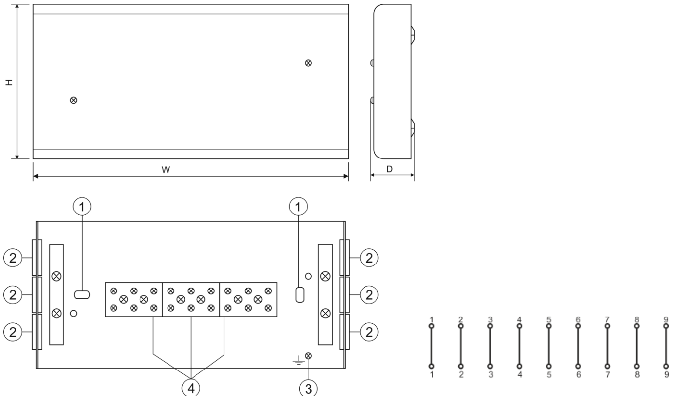
Rys.1. Widok puszki instalacyjnej.
