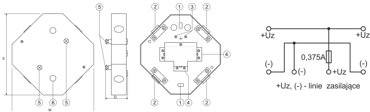
Rys.1. Widok puszki instalacyjnej i schemat połączeń.
