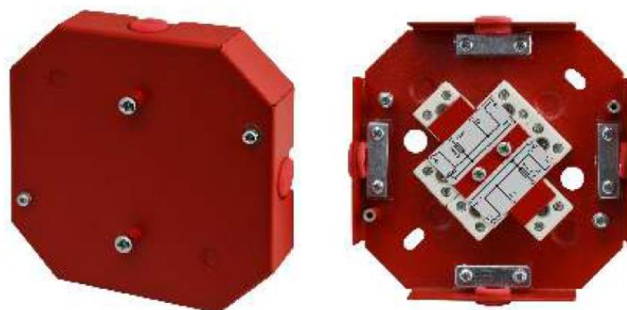
Ryc. 4. Puszka instalacyjna przeciwpożarowa typu AWOZ-225S. Źródło: Materiały producenta.
