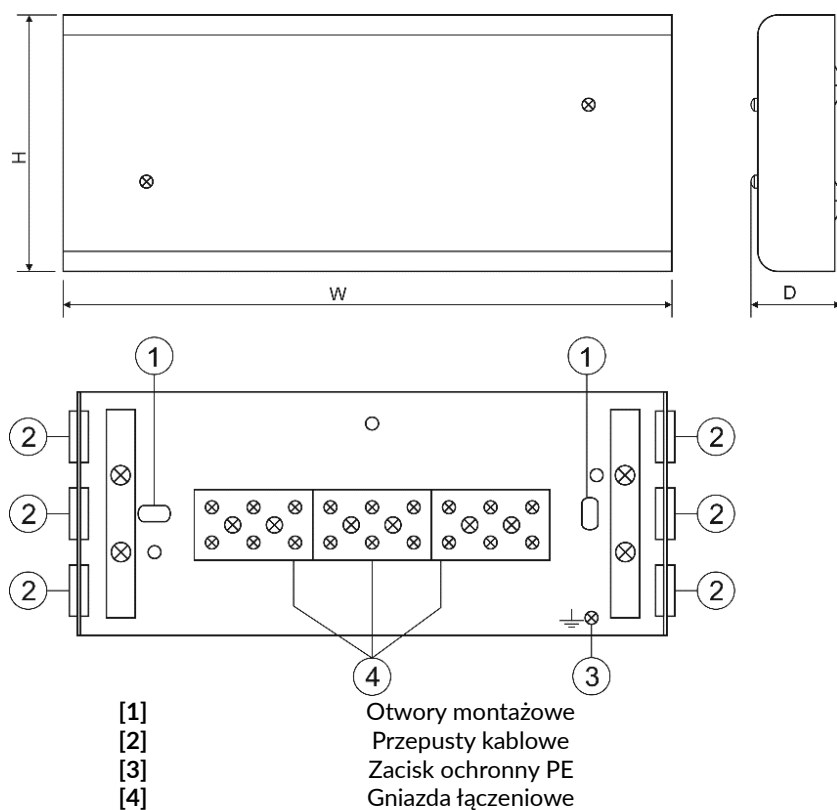
Ryc. 11. Puszka typu AWOP-925PP.
