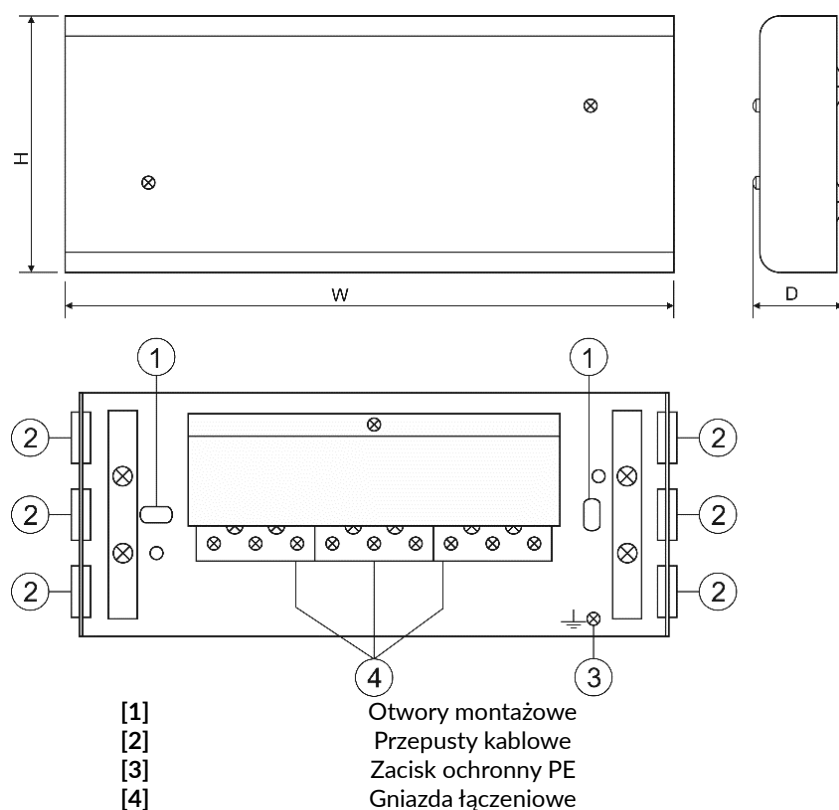
Ryc. 7. Puszka typu AWOP-325PR. Źródło: Materiały producenta.
