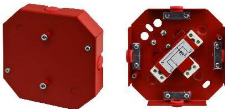
Ryc. 2. Puszka instalacyjna przeciwpożarowa typu AWOZ-125S. Źródło: Materiały producenta.
