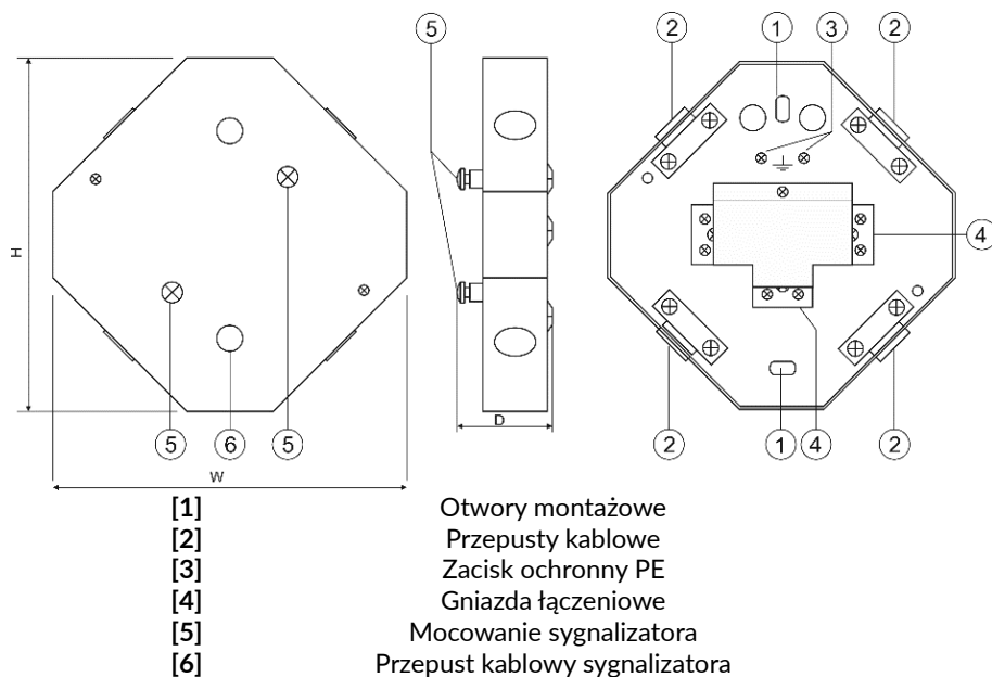
Ryc. 6. Puszka typu AWOP-225SR. Źródło: Materiały producenta.
