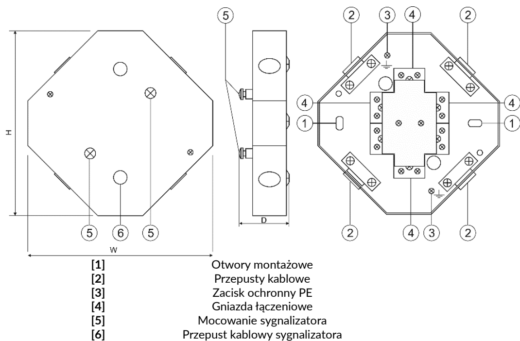
Ryc. 9. Puszka typu AWOP-425SR.
