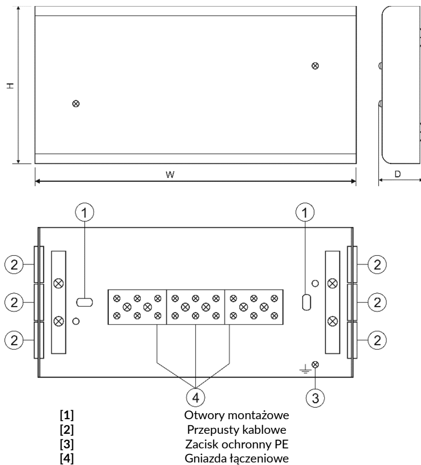
Ryc. 12. Puszka typu AWOP-960PP. Źródło: Materiały producenta.
