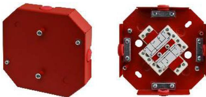
Ryc. 9. Puszka instalacyjna przeciwpożarowa typu AWOP-425SR. Źródło: Materiały producenta.
