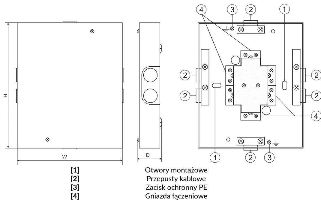
Ryc. 3. Puszka typu AWOZ-225P. Źródło: Materiały producenta.
