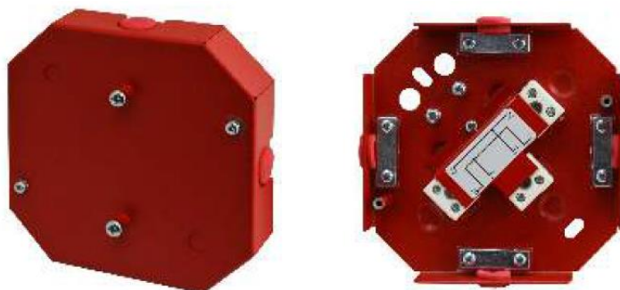
Ryc. 6. Puszka instalacyjna przeciwpożarowa typu AWOP-225SR. Źródło: Materiały producenta.
