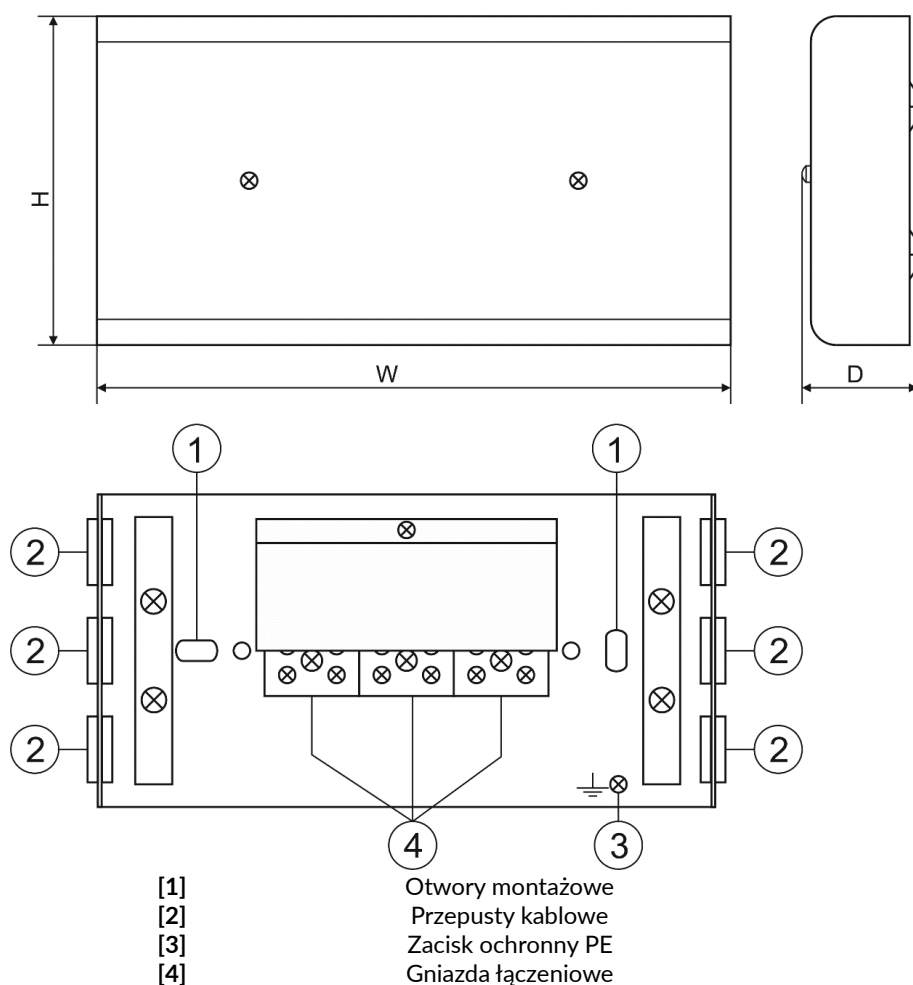
Ryc. 1. Puszka typu AWOZ-125P. Źródło: Materiały producenta.
