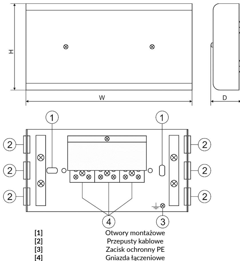
Ryc. 5. Puszka typu AWOP-225PR. Źródło: Materiały producenta.
