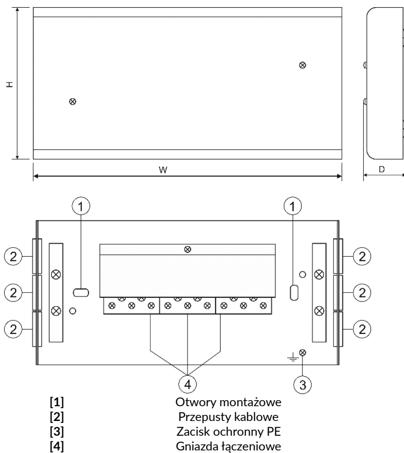
Ryc. 8. Puszka typu AWOP-360PR. Źródło: Materiały producenta.
