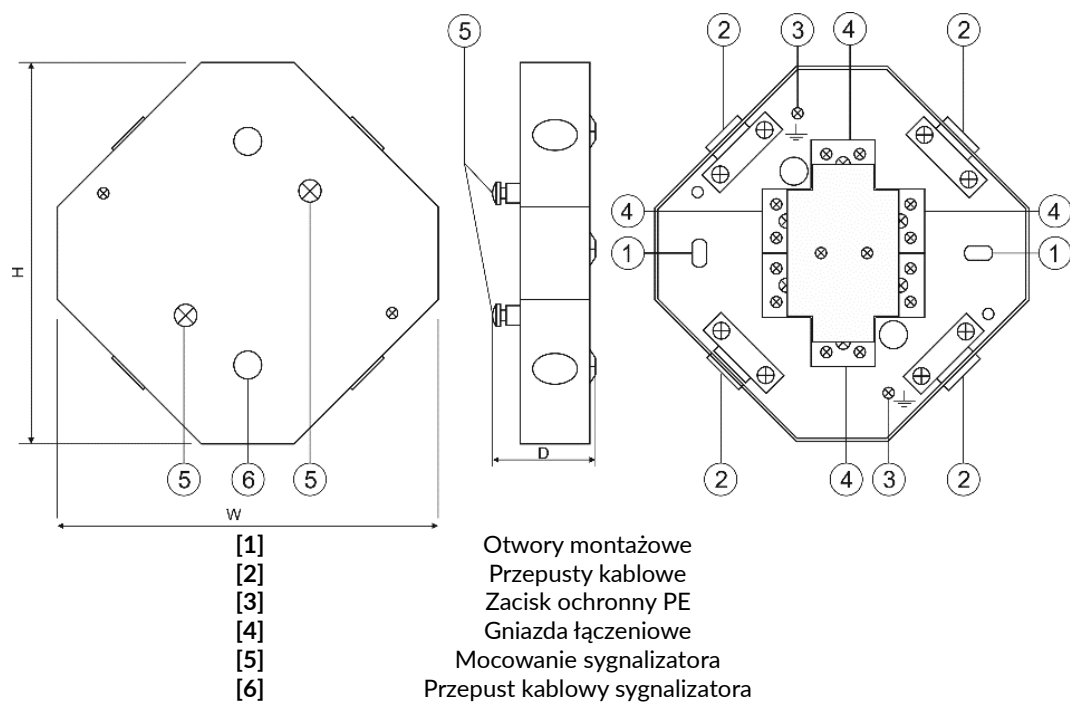
Ryc. 4. Puszka typu AWOZ-225S. Źródło: Materiały producenta.
