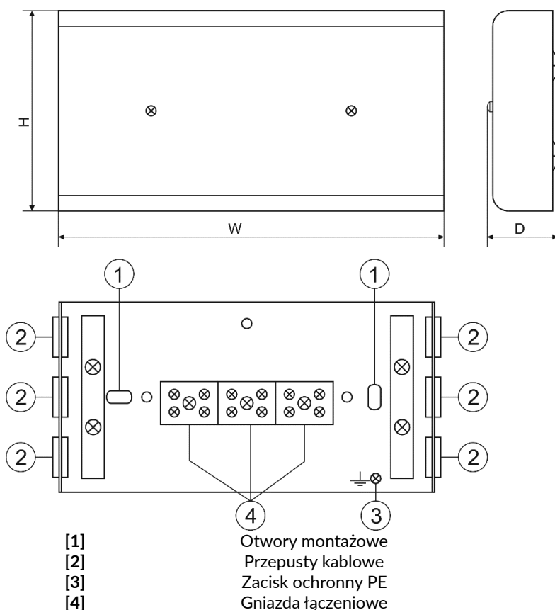
Ryc. 10. Puszka typu AWOP-625PP.
