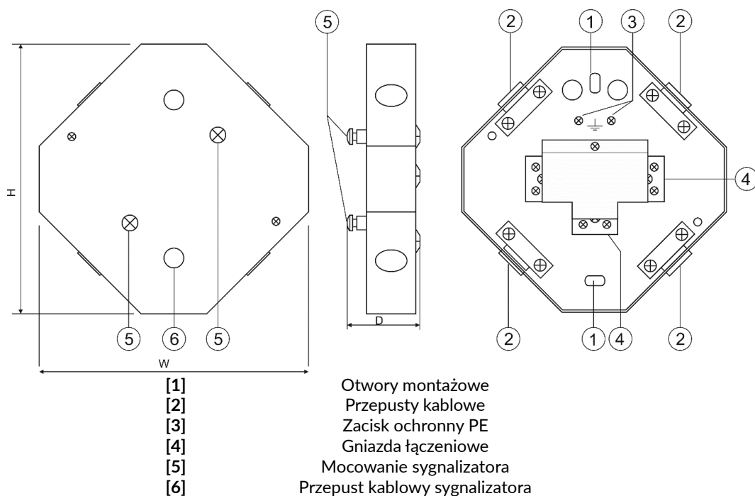
Ryc. 2. Puszka typu AWOZ-125S. Źródło: Materiały producenta.
